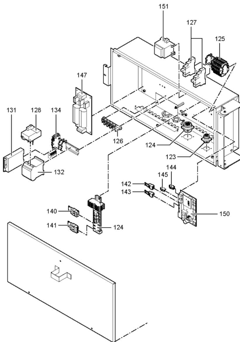
Anschlusskasten AWC-I und AW-O
