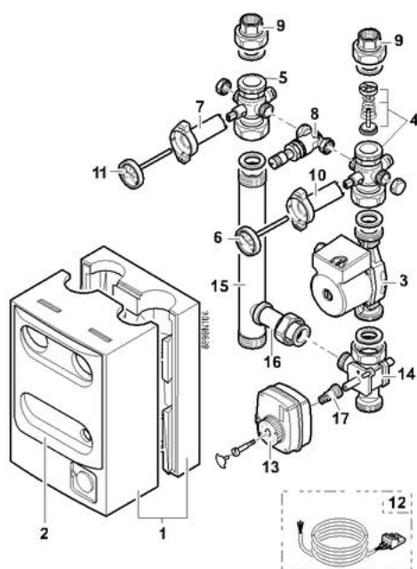
Module vanne 3 voies avec pompe électronique (Colis EA 68)
