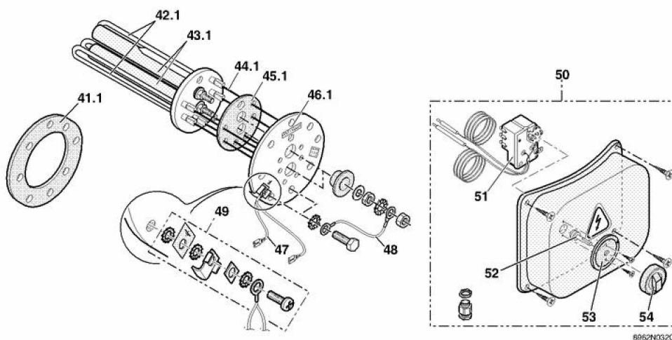
Résistances électriques 6.0 kW pour OB300-2 - OB400-2 - OB500-2 - OB300-2 B (options)
