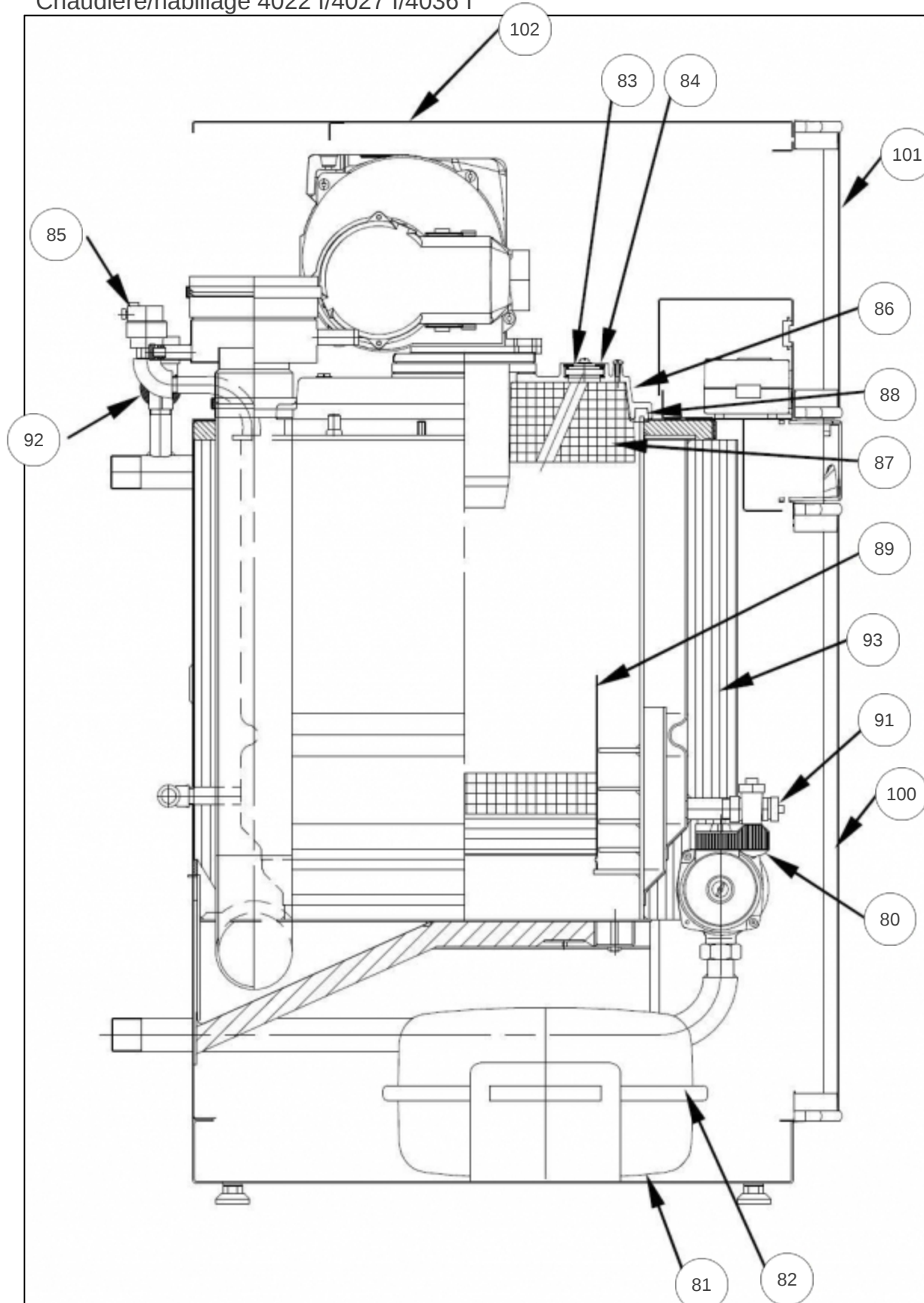
Chaudière/habillage 4022 I/4027 I/4036 I
