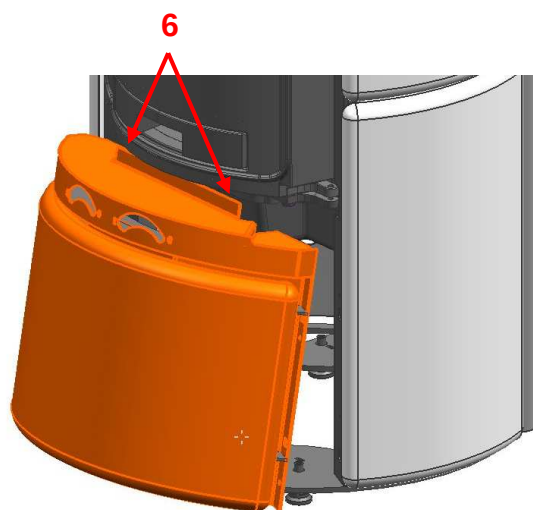
6 : Placer le tourne vis puis faire lever
