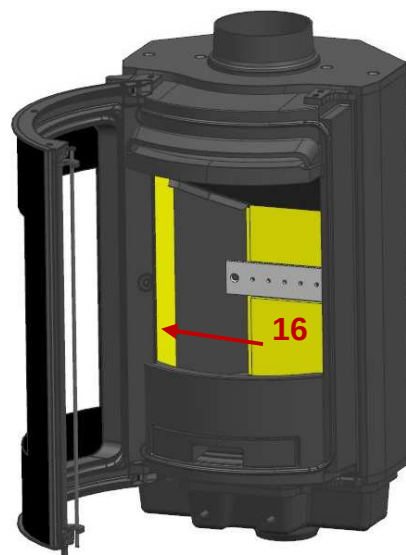
16 : Poser le réfractaire coté gauche sur la sole foyer et contre le coté gauche.
