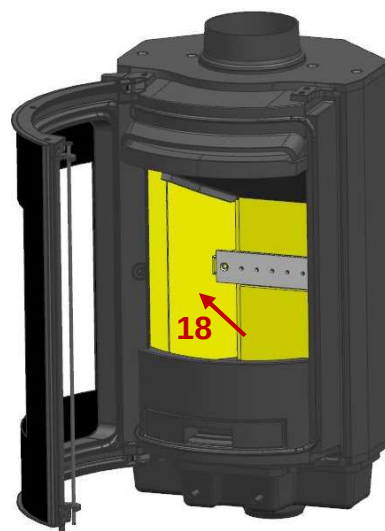
18 : Poser le réfractaire fond gauche sur la sole foyer et contre le fond.
