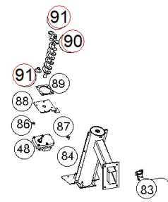
Assieme caricatore cod.249960
