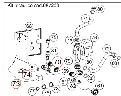
Kit Idraulico cod.687200
