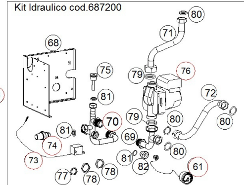
Kit Idraulico cod.687200
