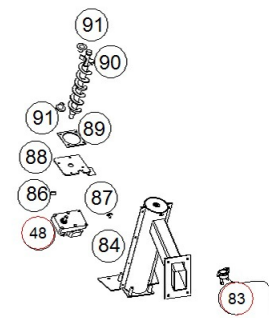
Assieme caricatore cod.24996C
