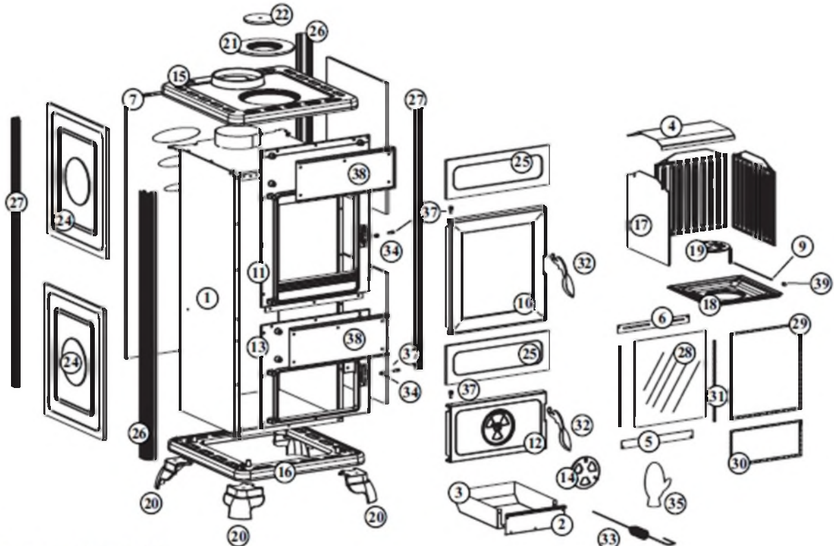
esploso GLORIA - ASIA
