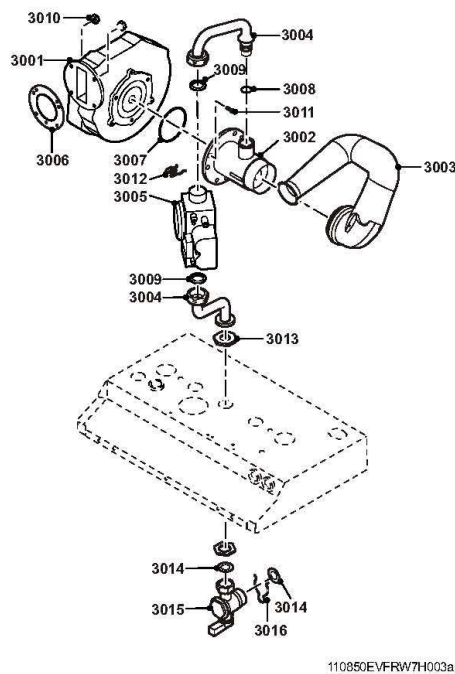
Ventilateur
