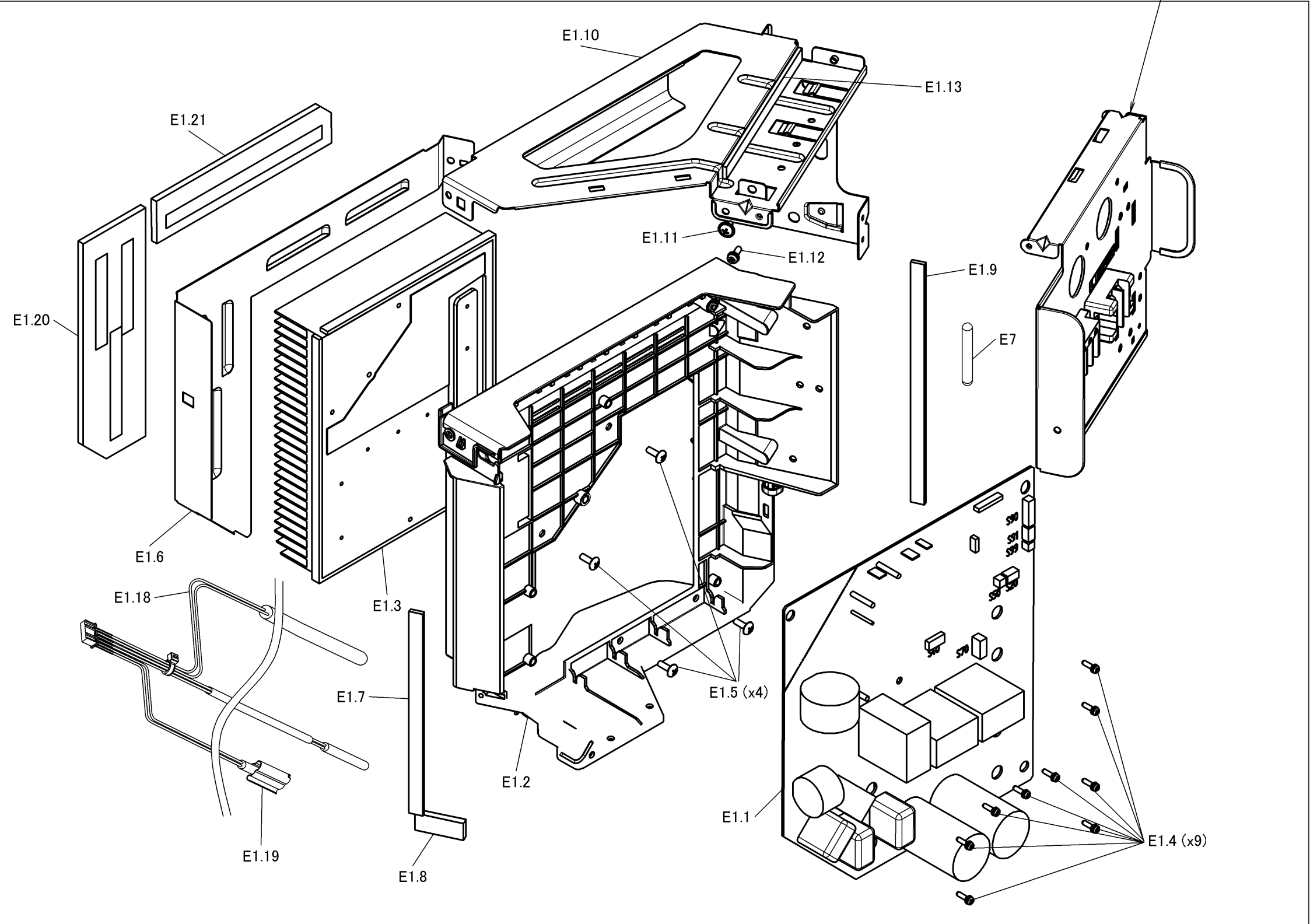
<E1: SWITCHBOX OUTDOOR UNIT>
