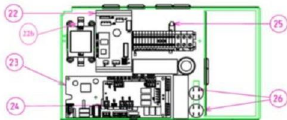
Détail - Composants platine électrique Detail - Electrical Panel Components
