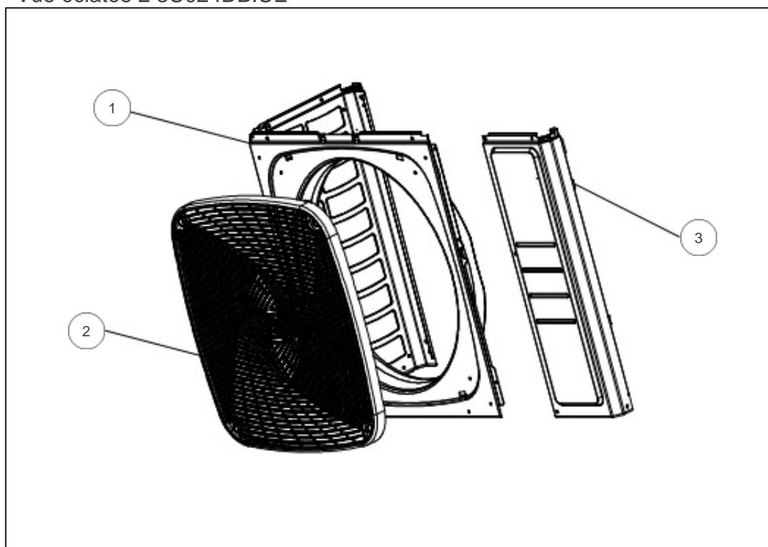
Vue éclatée 2 3U024DB.UE
