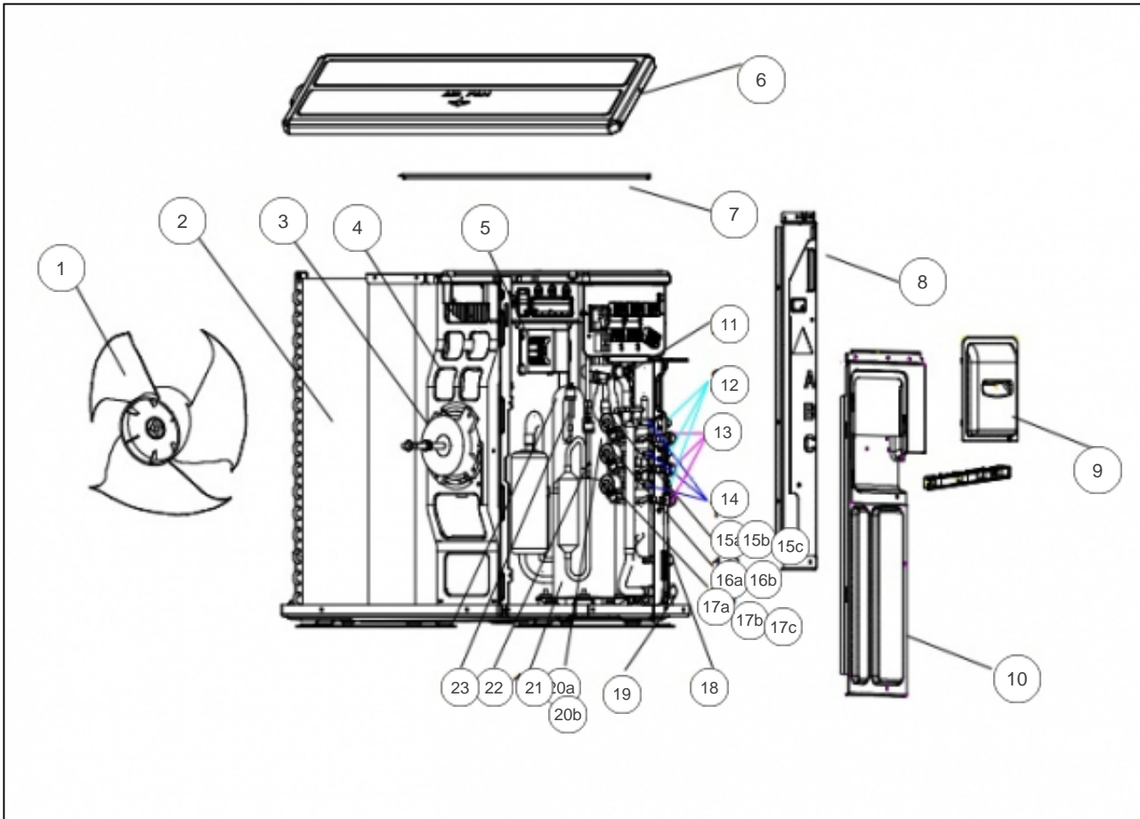
Vue éclatée 1 3U024DB.UE
