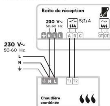
Chaudière combinée
