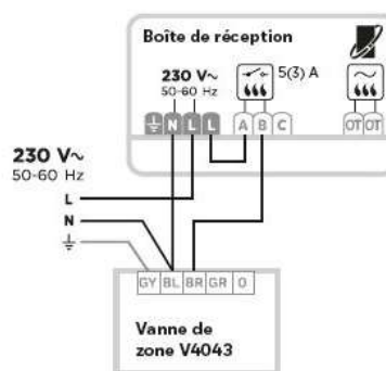
Vanne de zone à 2 ports
