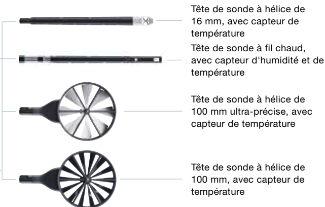
Têtes de sonde testo 440 pour les mesures de vitesse, avec capteur d'humidité et de température
